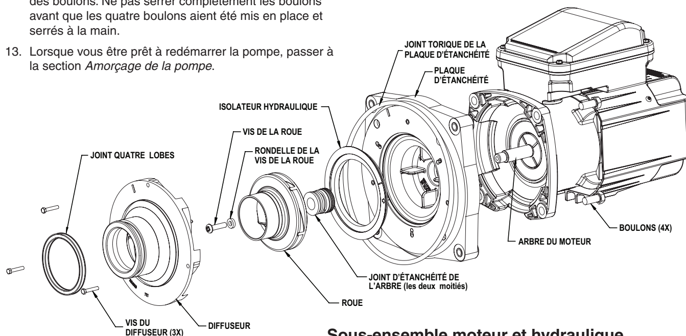
Sous-ensemble moteur et hydraulique
