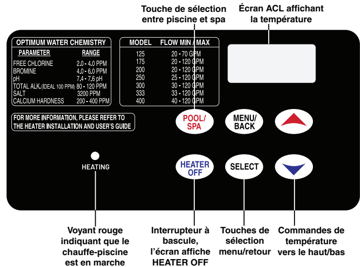
Figure 42. Panneau de commande du chauffe-piscine
