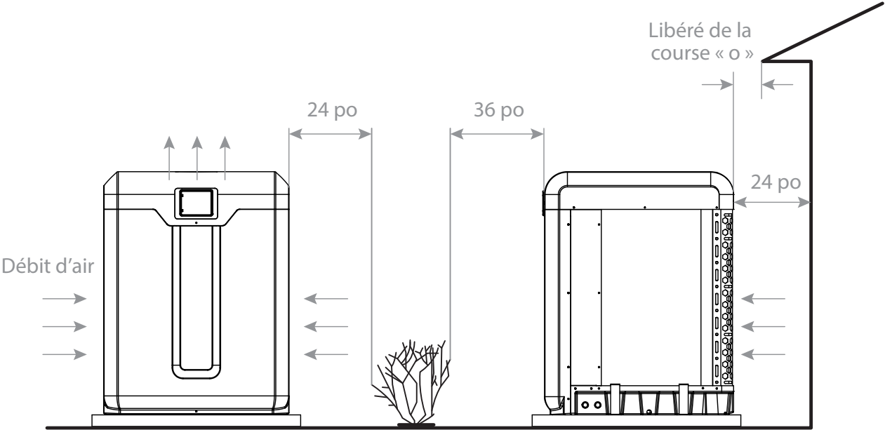
Figure 2 : Dégagements extérieurs minimums
