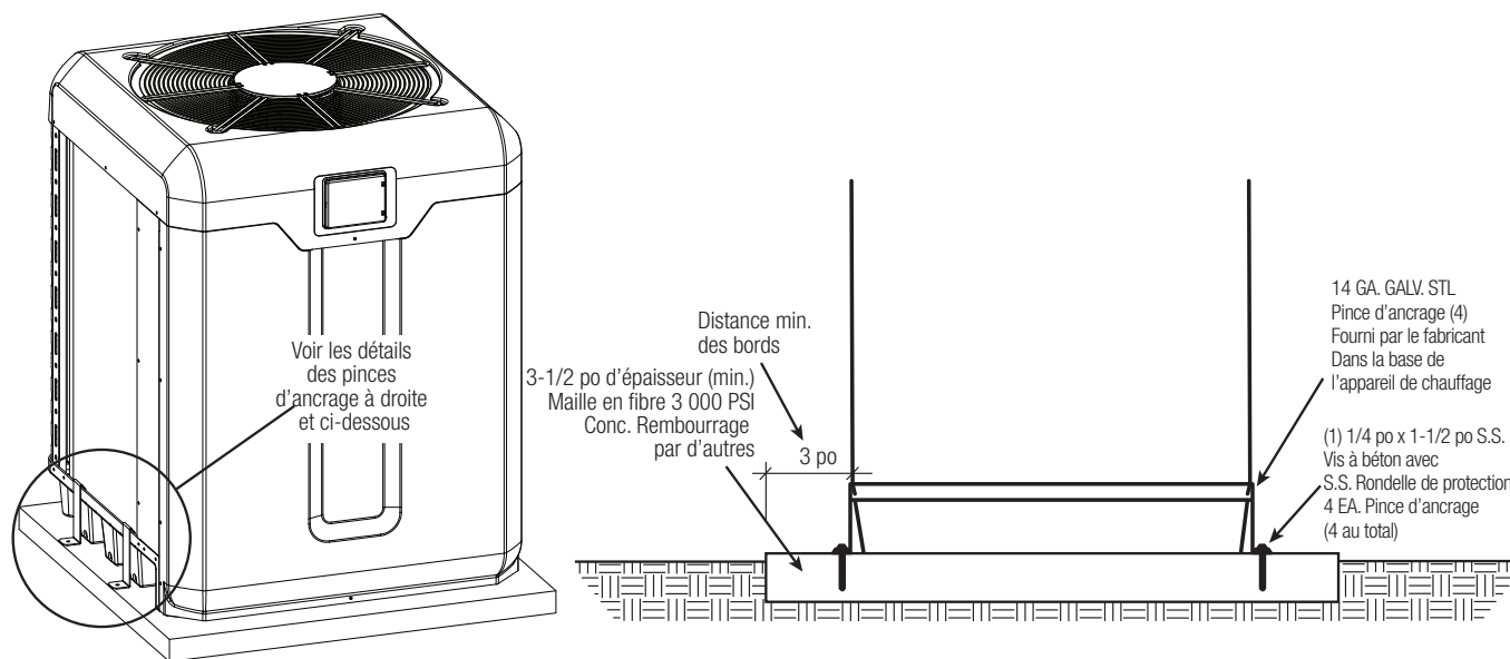
Figure 3 : Base Pour L'équipement et Ancrage
