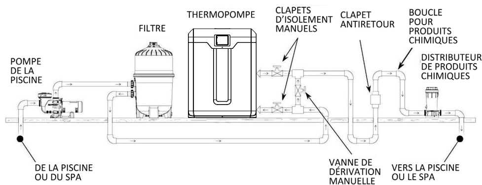
Figure 4 : Position Des Équipements Dans La Tuyauterie
