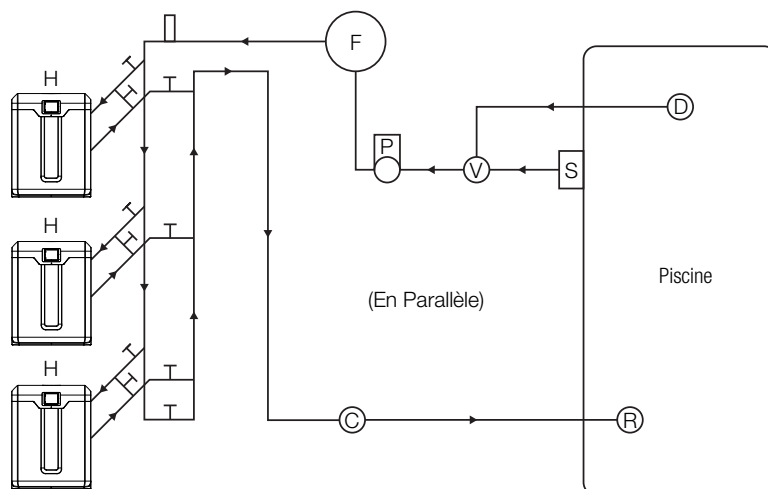
Figure 8 : Système à plusieurs thermopompes
