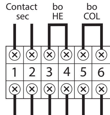
Figure 10 : Mise en marche / arrêt à distance
