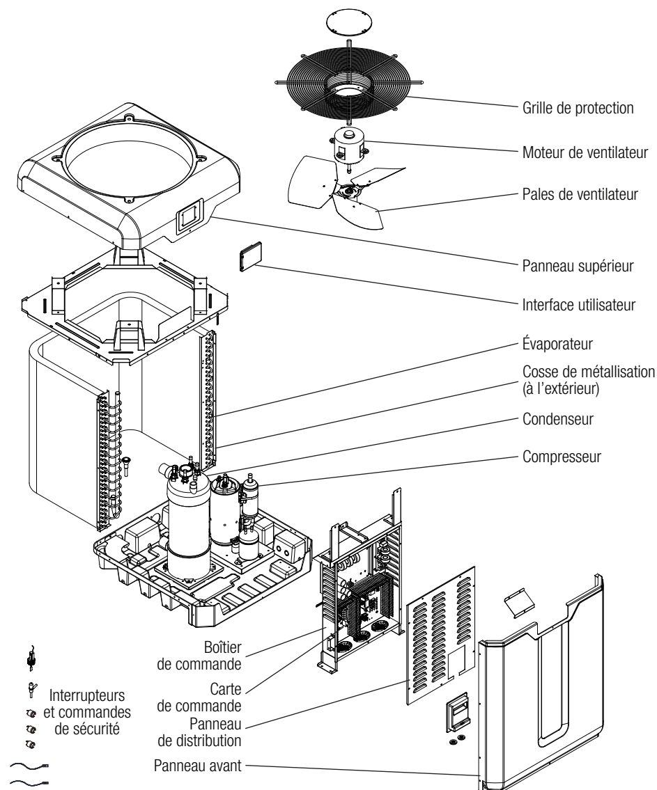
Figure 1 : Nom des composants de la pompe à chaleur
