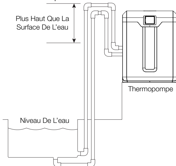
Figure 7 : Tuyauterie ordinaire vers la piscine
