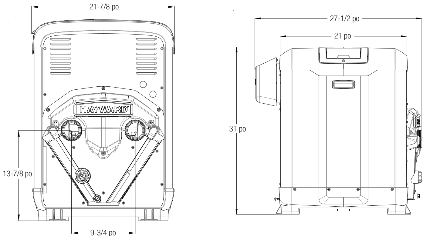
Figure 2 : Dimensions du chauffe-eau
