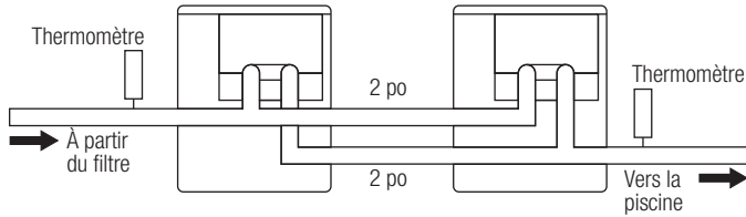
Figure 16 : Système à plusieurs chauffe-eau
