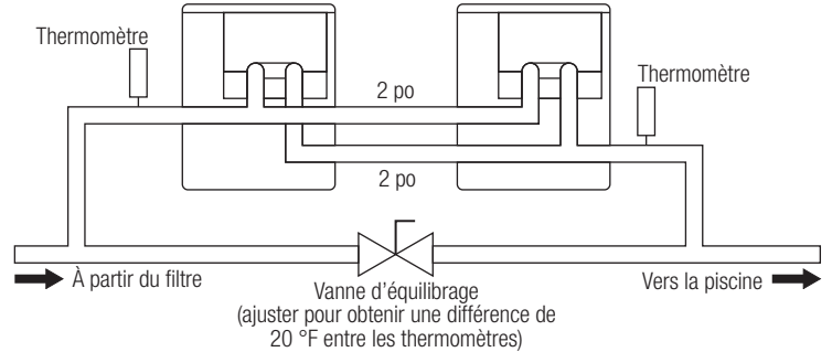
Figure 16 : Système à plusieurs chauffe-eau
