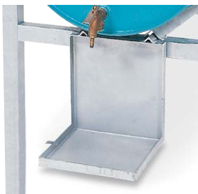
Support de récipient en acier, galvanisé Dimensions l x p x h : 280 x 270 x 300 mm N° de commande: 114-543-M2
