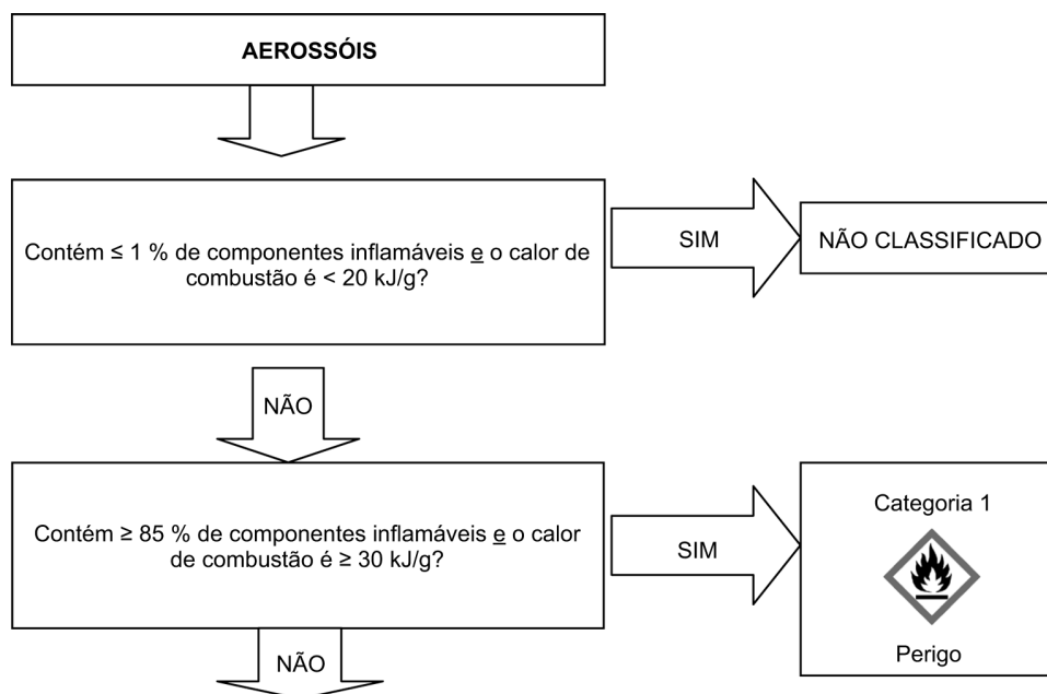
Figura 2.3.1 (a) aplicável aos aerossóis inflamáveis
