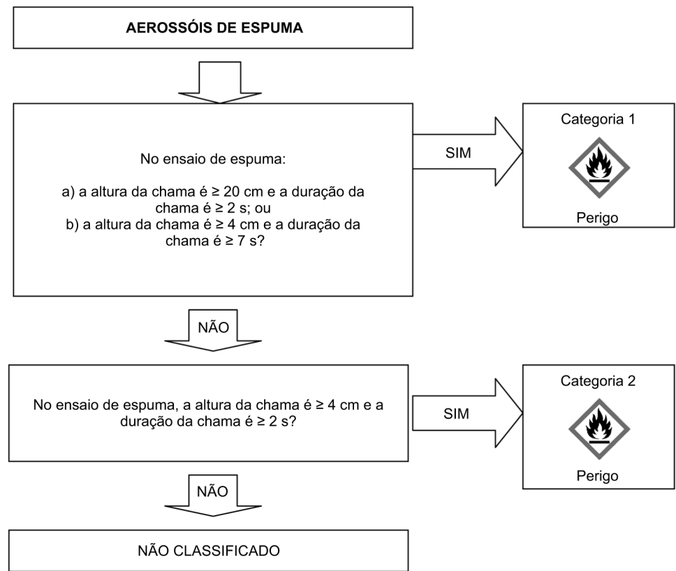
Figura 2.3.1 (c) aplicável aos aerossóis de espuma
