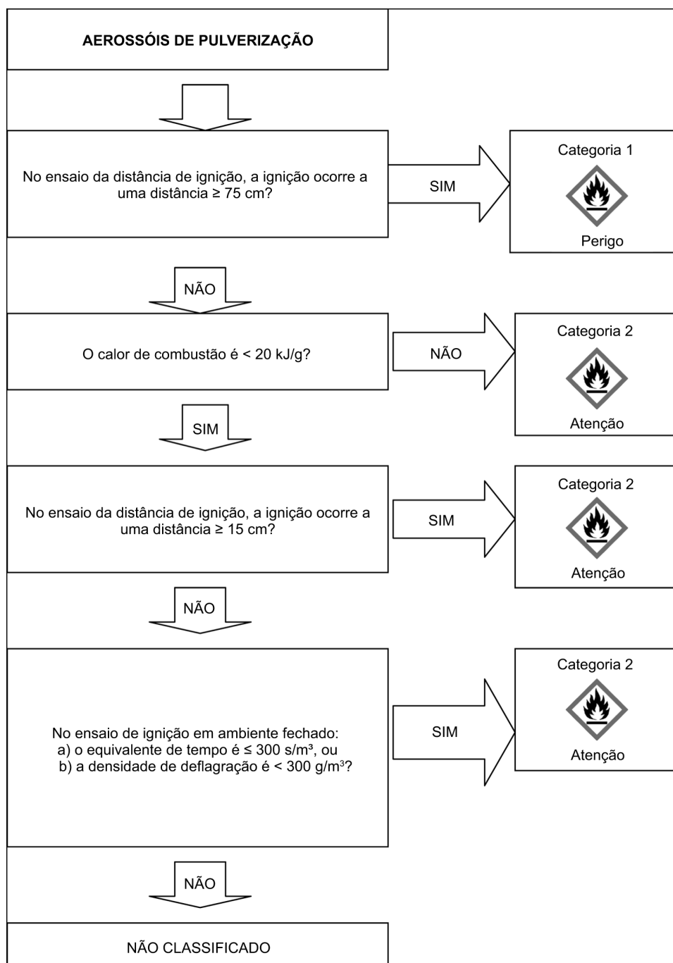
Figura 2.3.1 (b) aplicável aos aerossóis de pulverização
