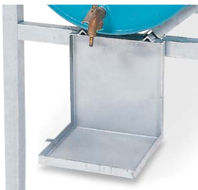
Stahl-Kannenträger, verzinkt Masse B x T x H : 280 x 270 x 300 mm Bestellnummer: 114-543-M2
