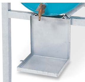
Support de récipient en acier, galvanisé Dimensions l x p x h : 280 x 270 x 300 mm N° de commande: 114-543-M2
