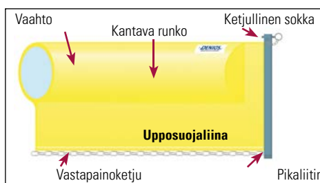
DENIOS-öljypuomin rakenne
