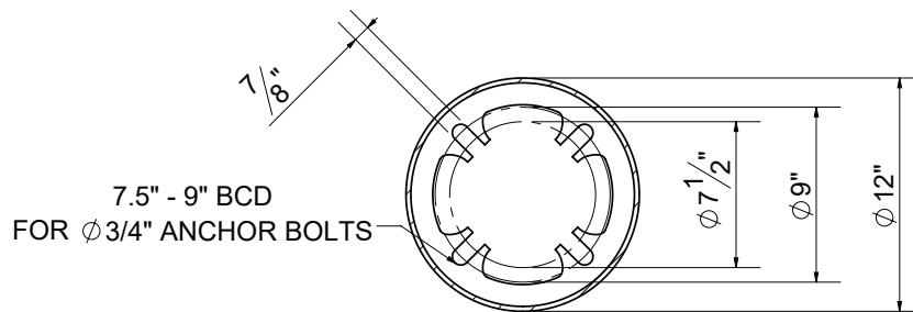
SECTION B-B SCALE 1 : 10
