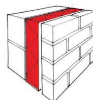
Gevelsteen in ecologisch formaat met meer isolatie
