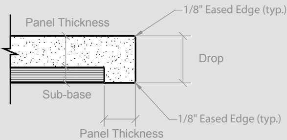
Drop Down Edge
