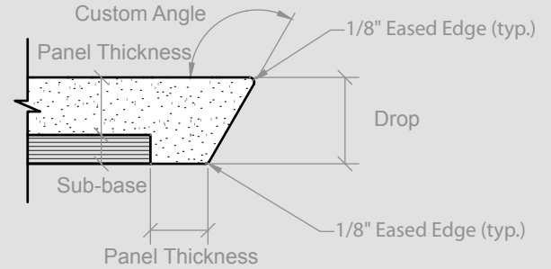
Drop Down Mitered Edge
