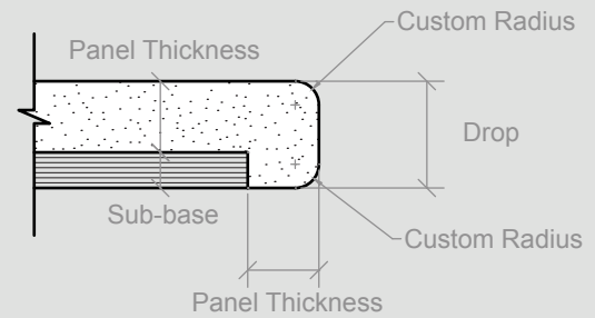
Drop Down Radiused Edge
