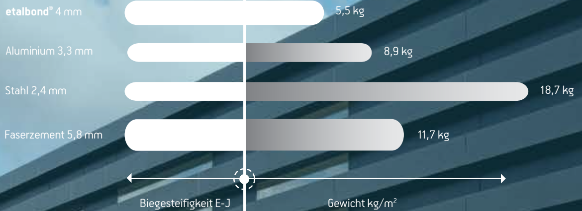
Vergleich von Dicke und Gewicht bei identischer Biegesteifigkeit
