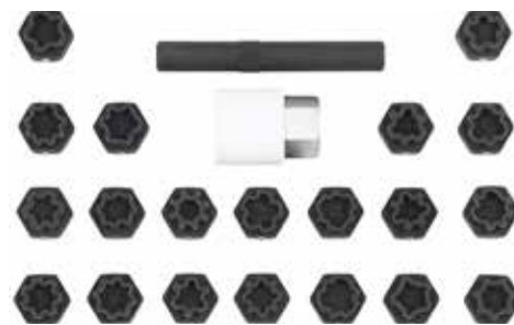
#829006 Coffret débloccage écrous antivol, 22-pcs Kit complet comprenant un adaptateur 1/2" de 21mm. Permet d'enlever les écrous antivol en l'absence de l'adaptateur fourni par le constructeur.
