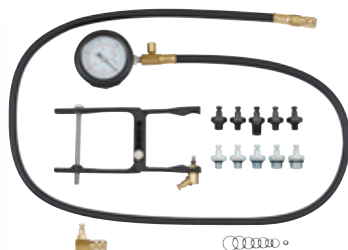
#818011 Coffret testeur pression d'huile, 14-pcs
