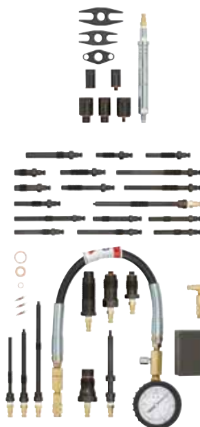
#818010 Coffret testeur de compression essence et diesel, 37-pcs
