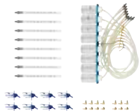
#818009 Coffret contrôle de retour d'injecteurs common rail 8 cylindres, 31-pcs
