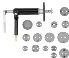
#801016 Coffret repousse pistons pneumatique pour étriers de freins, 16-pcs
