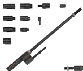
#829003 Extracteur pneumatique d'injecteurs diesel Permet de retirer les injecteurs de la culasse. Equipé d'un filetage mâle 5/8" pour la con- nection à tout adaptateur de marteau à inertie.
