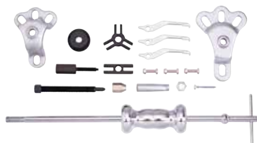
#808001 Coffret extracteurs de moyeux à inertie, 16-pcs
