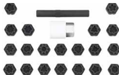
#829006 Coffret déblocage écrous antiviol, 22-pcs Kit complet comprenant un adaptateur 1/2" de 21mm. Permet d'enlever les écrous antiviol en l'absence de l'adaptateur fourni par le constructeur.
