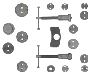
#801018 Coffret repousse pistons manuel pour étriers de freins, 18-pcs
