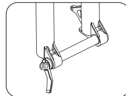
Steckachse in den Gabelausfallenden, ohne Nabe, Rock Shox® Gabel
