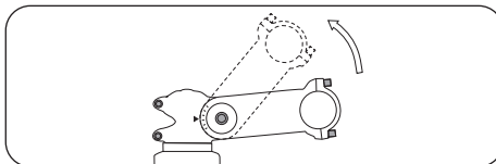
Verstellung der Vorbau-Neigung möglich
