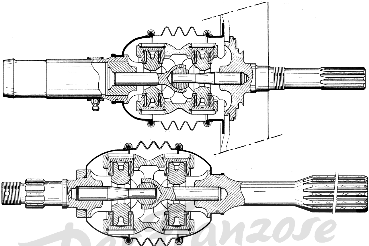
Schnitt durch ein homokinetisches Doppelkreuzgelenk
