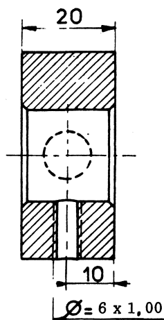
Schnitt B
