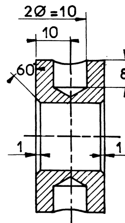
Schnitt A
