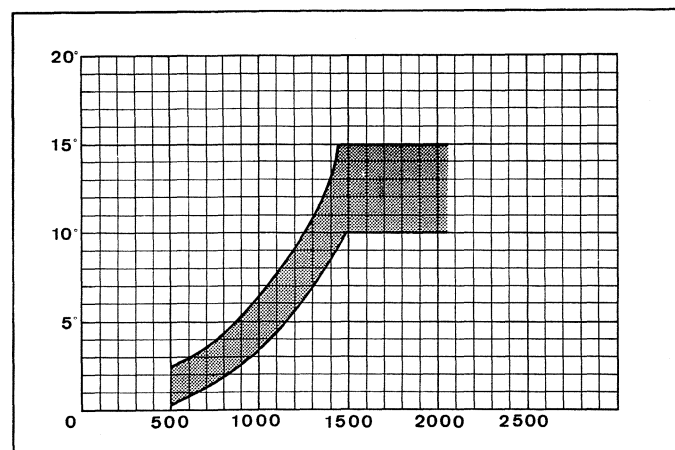
Verstellkurve C
