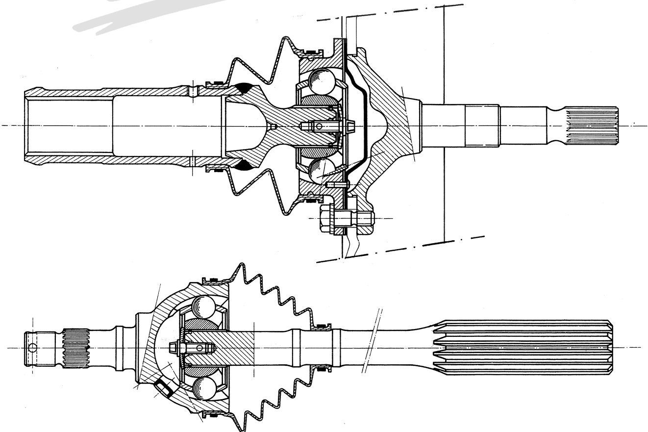
Schnitt durch ein homokinetisches Kugelgelenk
