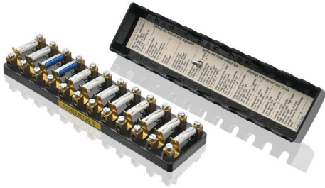
Boîte à fusibles 12 fusibles Réf. 90161280120 911 type F (1965–1968)
