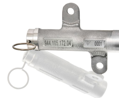
Amortiguador tensor de correa N.º referencia: 94410517204 968 (1992–1995)
