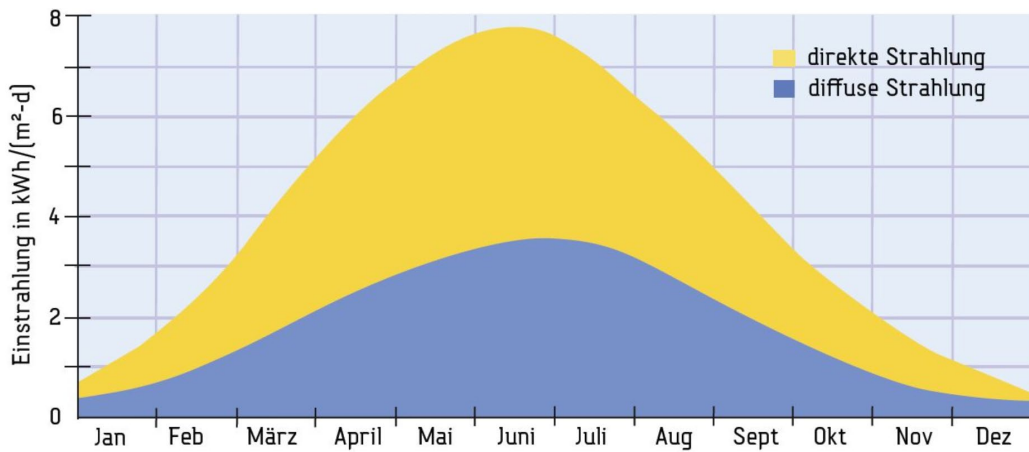
Abbildung 40: Verlauf der Einstrahlung der Sonne während eines Jahres 51
