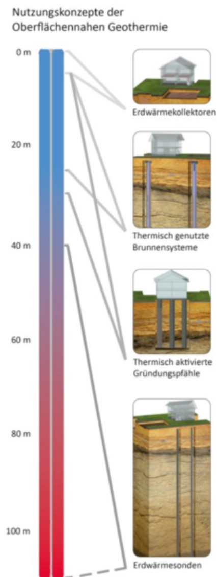
Abbildung 38: Darstellung der oberflächennahen Geothermie – vgl. 39
