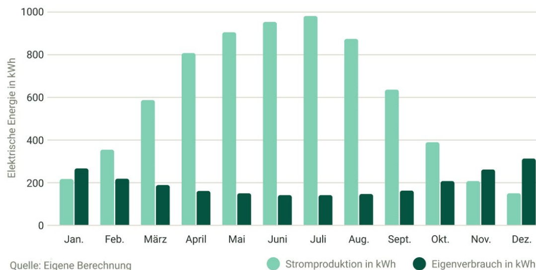
Abbildung 52: Beispielhafte Grafik einer Stromproduktion und Eigenverbrauch eines Einfamilienhauses mit einer 7.000kWp PV-Anlage und einem eigenen Stromverbrauch von 2.500kWh 76
