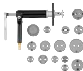
#801016 Remzuiger terugstel gereedschapset pneumatisch, 16-dlg.
