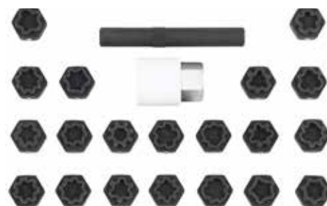
#829006 Wielmoersleutelset - geschikt voor Audi, 22-dlg. Compleet met 21mm adapter met 1/2" aansluiting vierkant. Deze set is bedoeld voor het verwijderen van slotbouten als de klant is vergeten de originele dop bij de auto te leveren. Komt overeen met OEM T40073.
