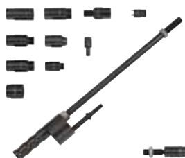
#829003 Verstuiver-slagtrekker voor pneumatische hamer Onmisbare set om op professionele wijze vastzittende inspuitsstukken te verwijderen uit de cilinderkop.
