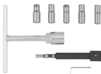
#818004 Frezen voor verstuiverzittingen en brand-plaatjesset, 7-dlg.
