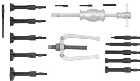
#818021 Lager trekkerset, 16-dlg.
