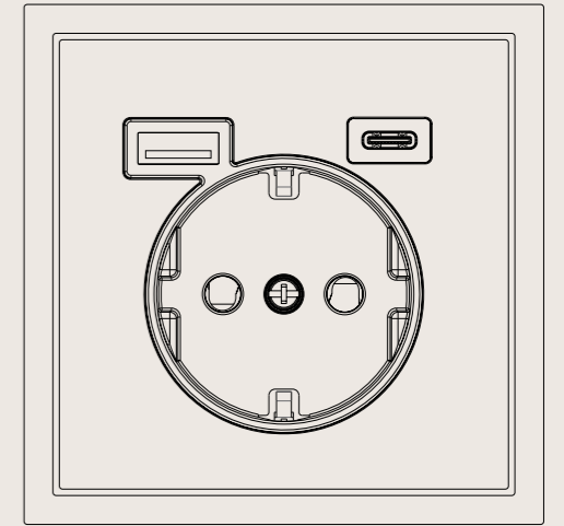
BASE + USB A+C SOCKET + USB A+C
