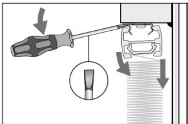
Falzmontage Top fixing Montage en feuillure Montaggio a libro
