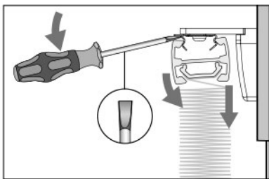
Winkelmontage Face fixing Montage en angle Montaggio ad angolo
