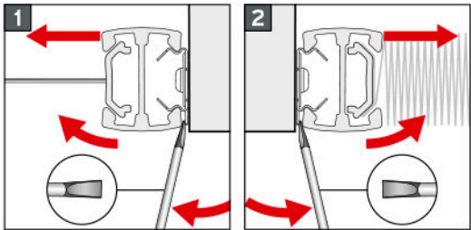
Falzmontage Top fixing Montage en feuillure Montaggio a libro
