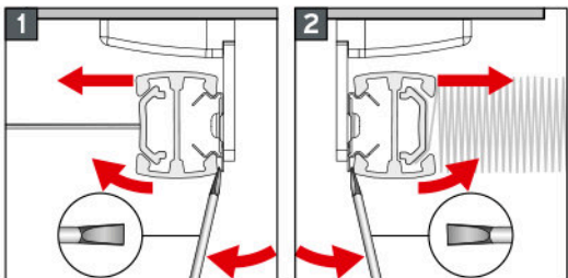
Winkelmontage Face fixing Montage en angle Montaggio ad angolo
