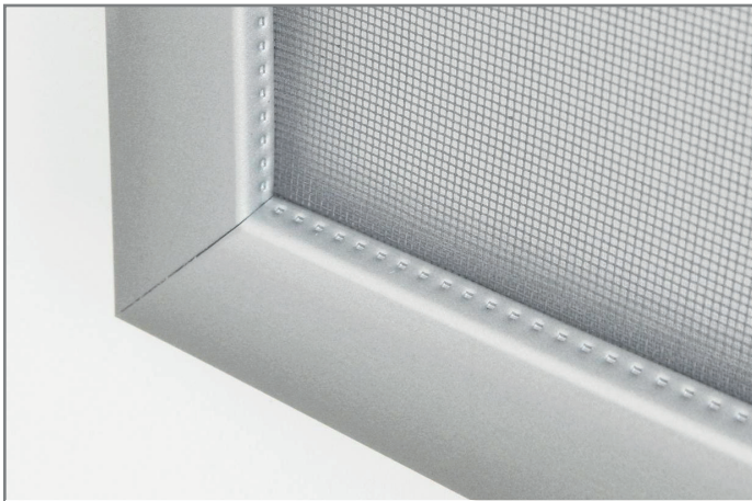
Die Rahmenecken sind auf Gehrung geschnitten
