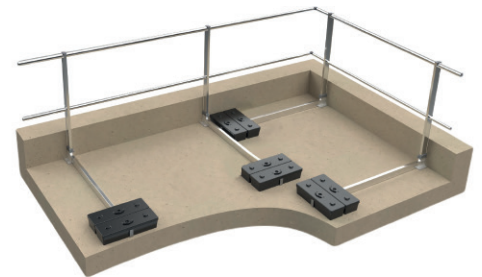
Geländersysteme
