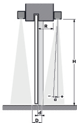
Schnitt durch Schiebetür, beidseitig mit Sensoren und gegenüberliegenden AIR-Feldern
