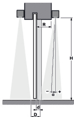
Doorsnede schuifdeur, aan beide zijden met sensoren en tegenoverliggende AIR-velden
