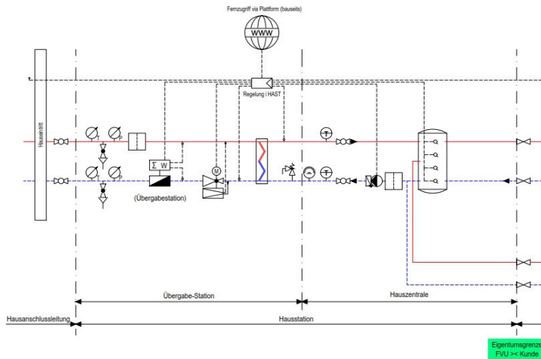
Abbildung 3: Grenzen nach Typ 2 (Fernwärme-Hausanschluss Plus)
