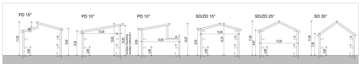
Beispielhafte Systemschnitte zur Darstellung der festgesetzten maximalen Trauf- und Gebäudehöhen im WA2 bei verschiedenen Dachformen, FSP (ohne Maßstab)
