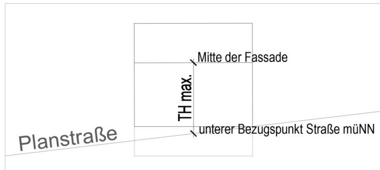
Beispielhafte Schemaskizze zur Darstellung der Bemessung des unteren Bezugspunktes und der festgesetzten maximalen Traufhöhen, FSP (ohne Maßstab)
