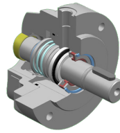
Gleitringdichtung mit Radialwellendichtring und Anschlussbohrung für Flüssigkeitsvorlage
