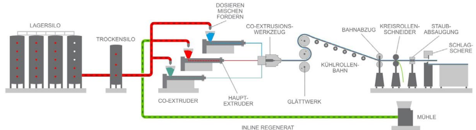
Abb. 4: Extrusionsprozess
