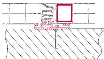
Flachsoganker / Verstärkungsrohr
