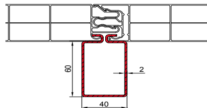
Stahl-Versteifungsprofil
