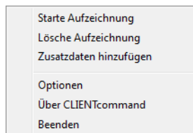
Abb. 11: Zusatzdaten hinzufügen
