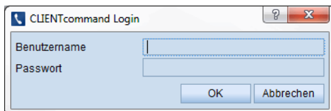
Abb. 2: Login-Fenster
