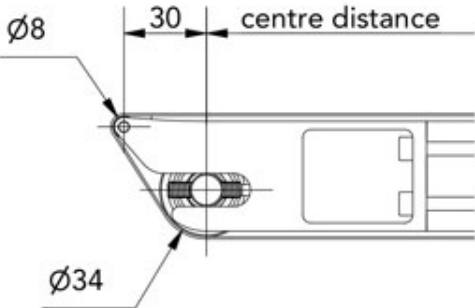
Knife edge
