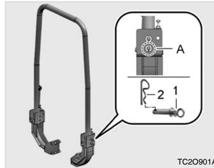
(1) Befestigungsstift (2) Clip-Stift
