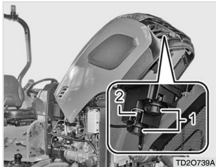
(1) Kappe
