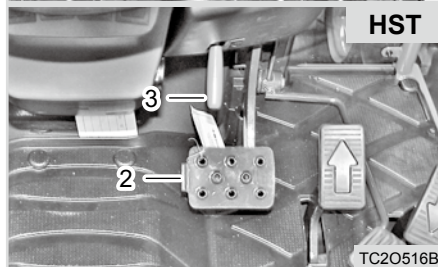
(1) Block (2) Parkbremse (3) Parkbremshebel (4) Parkbremspedal
