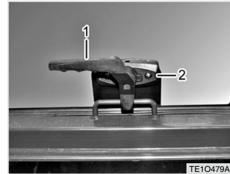
(1) Griff des Heckfensters (2) Sperrvorrichtung
