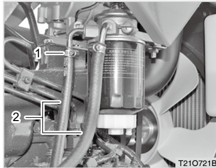
(1) Kraftstoffleitung (2) Kraftstoff-Schlauchklemmen
