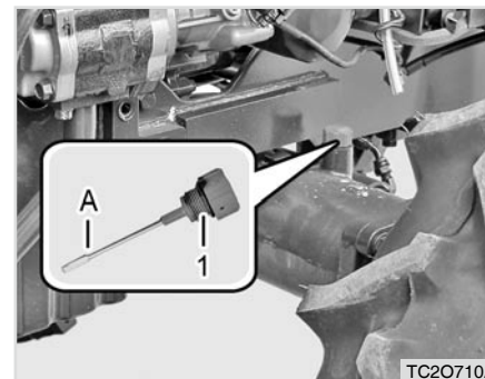
(1) Ölstab
