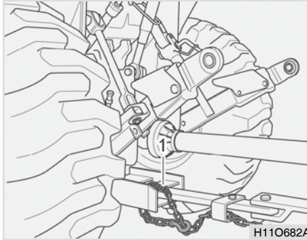
(1) Sicherheitskette
