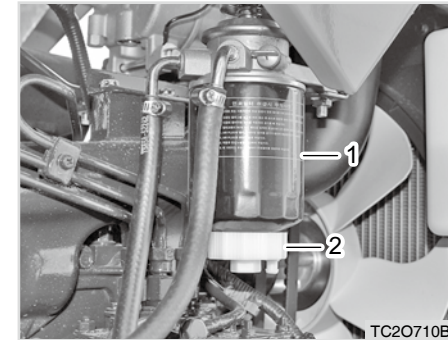
(1) Kraftstofffilter (2) Ölablassschraube
