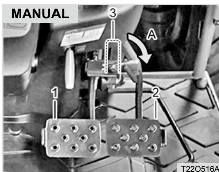
(1) Bremspedal (L) (2) Bremspedal (R) (3) Riegel der Pedalverriegelung (A) Beim Befahren von Straßen
