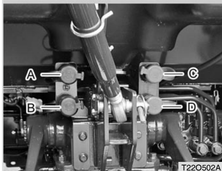
(1) Hebel für zweifachwirkendes Ventil 1 & Hebel 1 (2) Hebel für zweifachwirkendes Ventil 2 & Hebel 2 (A) Anschluss A (B) Anschluss C (C) Anschluss B (D) Anschluss D
