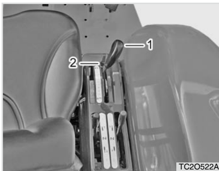
(1) Positionskontrollhebel (2) Sperrbolzen
