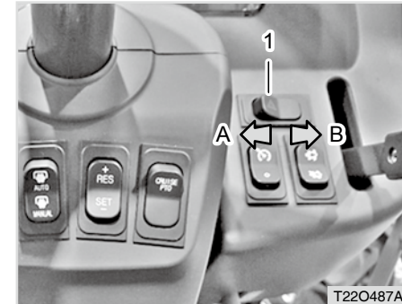
(1) Warnblinkschalter (A) EIN (B) AUS
