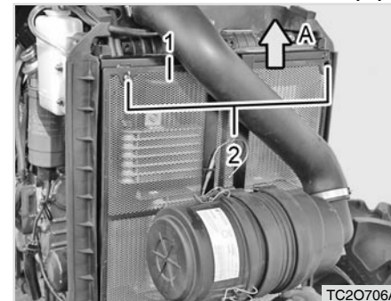
(1) Ölkühlergitter (A) Entfernen
