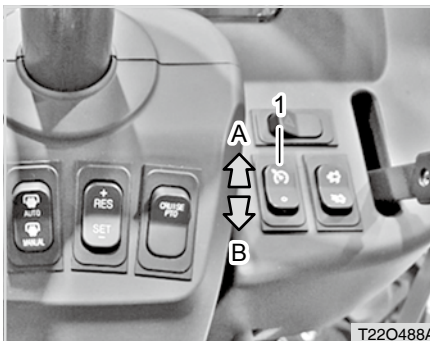
(1) Kontrollschalter Zapfwellen-Geschwindigkeitsregler
