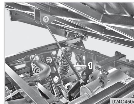
(1) Hydraulikzylinder
