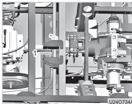
(1) Feststellbremskabel
