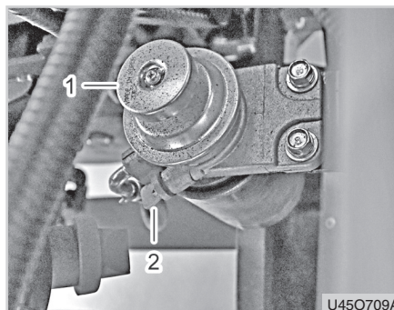
(1) Antriebspumpe (2) Entlüftungstopfen
