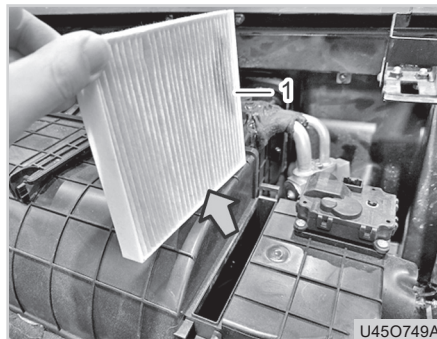
(1) Verschmutzter Filter
