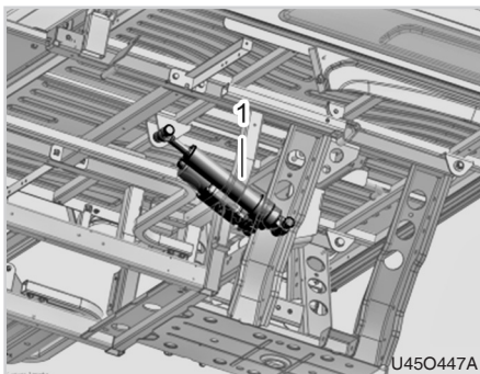
(1) Hubzylinder
