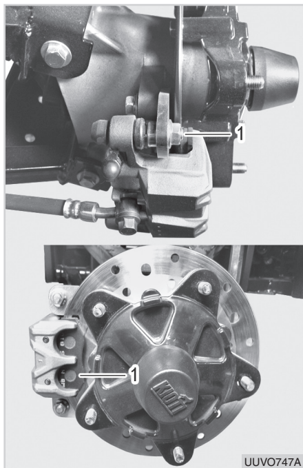
(1) Bremsbacke
