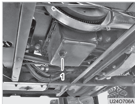
(1) Ablaßschraube
