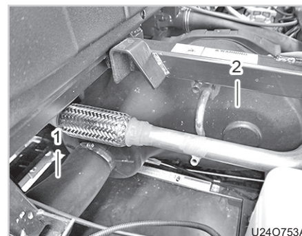
(1) Luftschlauch (2) CTV-Abdeckung
