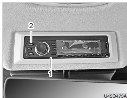
(1) Bluetooth-Spieler/Radio (2) Netzschalter
