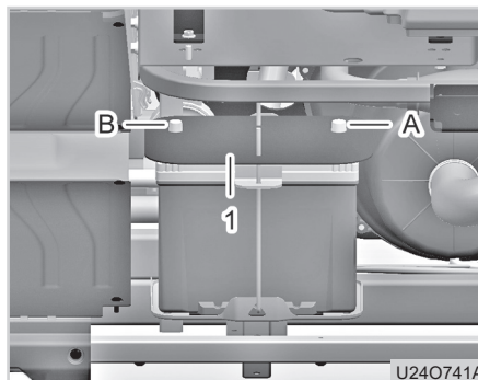
(1) Batterieabdeckung (A) Plus (+) Kabel (B) Minus (-) Kabel
