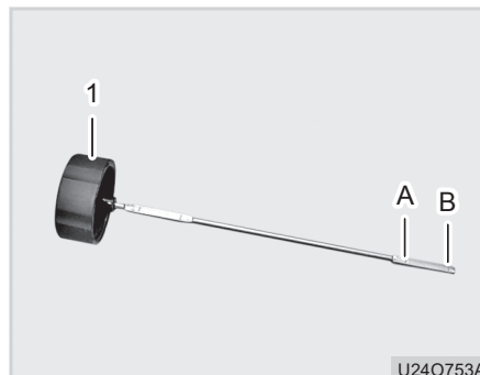
(1) Ölmesstab (A) Grenze MAX (B) Grenze MIN
