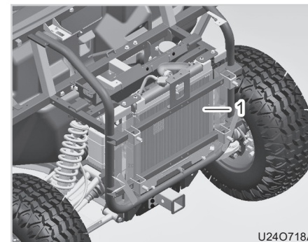
(1) Kühler
