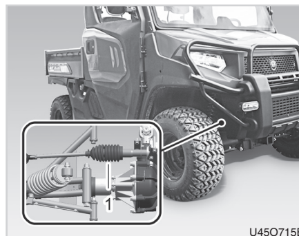
(1) Schutzhülle am Lenkgestänge
