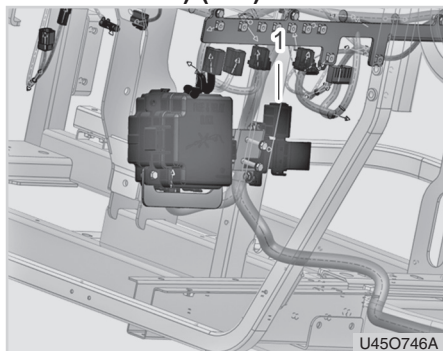
(1) Träge Sicherung
