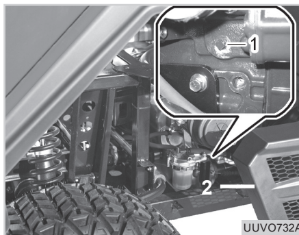
(1) Kühlflüssigkeit-Ablaßschraube (2) Motorölfilter
