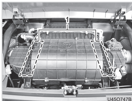
(1) Klimaanlagefilter-Abdeckung
