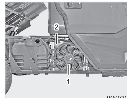
(1) Kühlgebläse (2) Kondensator
