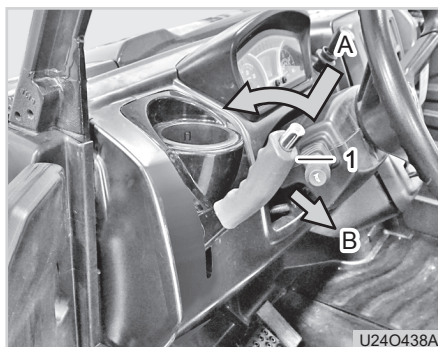
(1) Feststellbremse
