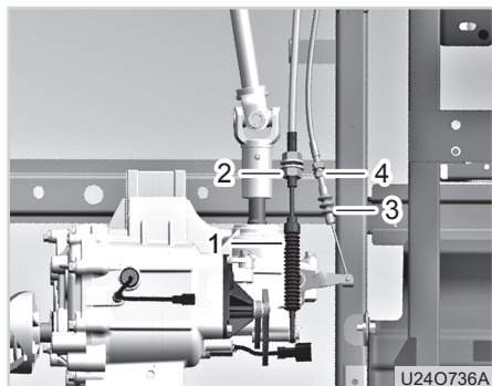
(1) Getriebekabel (2) Mutter 1 (3) Allradantriebskabel (4) Mutter 2
