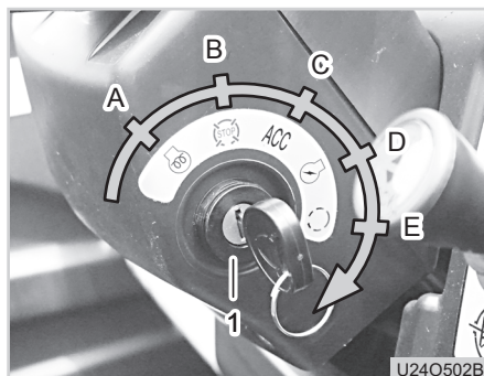
(1) Schlüsselschalter (A) AUS (B) ACC (C) EIN (D) Vorwärmen (E) Start
