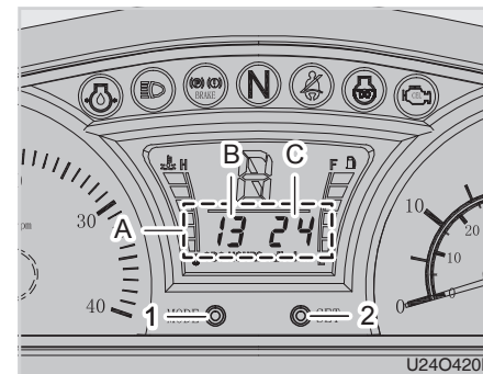
(1) Moduswahl-taste (2) Set-Taste (A) Stundenzähler (B) Stundenanzeige (C) Minutenanzeige
