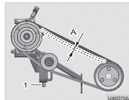
(1) Einstellbolzen
