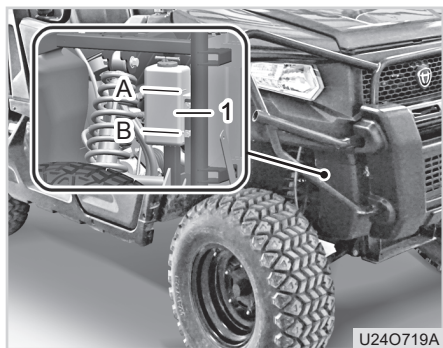
(1) Ausgleichsbehälter (A) MAX Markierung (B) MIN Markierung
