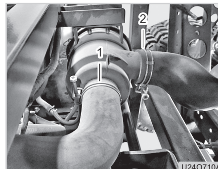
(1) Klemme 1 (2) Klemme 2
