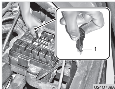
(1) Sicherungszange
