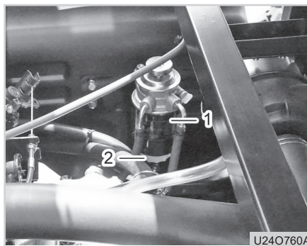
(1) Kraftstofffilter (2) Ölablassschraube
