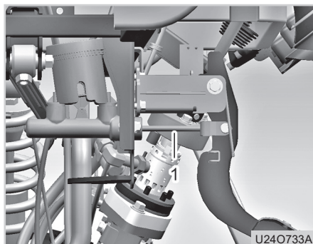
(1) Hauptzylinderstange
