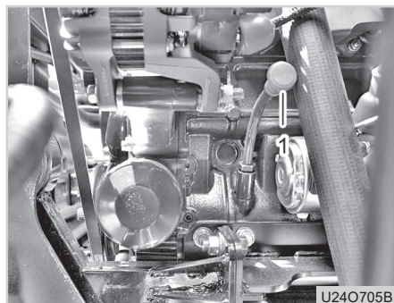
(1) Ölpeilstab
