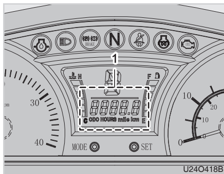
(1) Stundenzähler, Wegstreckenzähler
