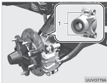
(1) Schmiernippel
