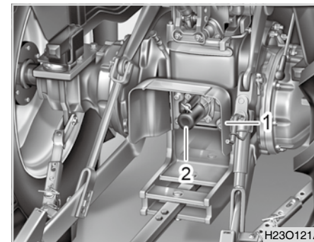
(1) Zapfwellenabdeckung (2) Zapfwellendeckel
