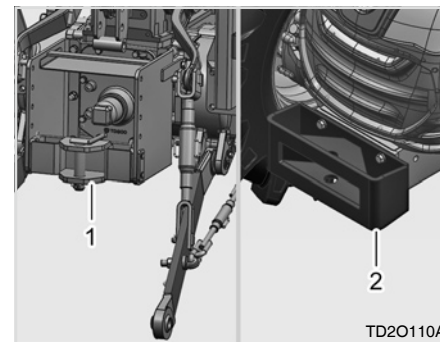
(1) Zugstange
