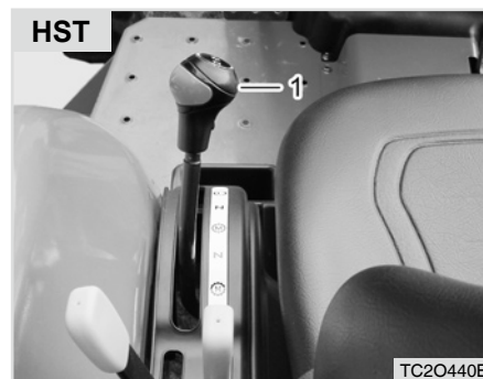
(1) Bereichsschalthebel
