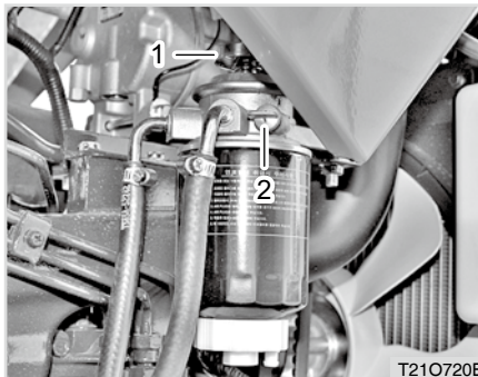
(1) Antriebspumpe (2) Entlüftungsschraube
