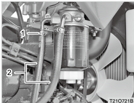
(1) Kraftstoffleitung
