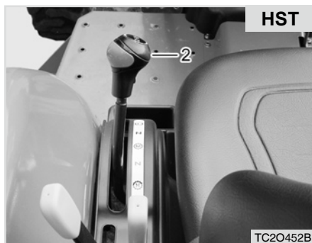
(1) Hauptschalthebel (2) Bereichsschalthebel
