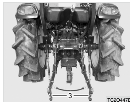
(1) Positionskontrollhebel (2) Sperrbolzen (3) Unterer Lenker (A) Senken (B) Heben
