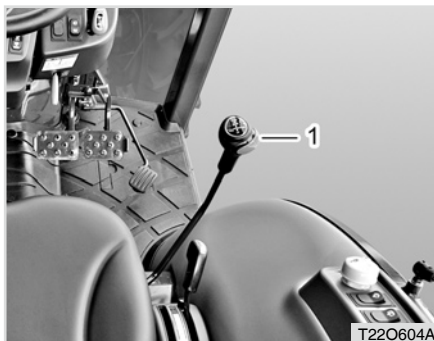
(1) Steuerhebel
