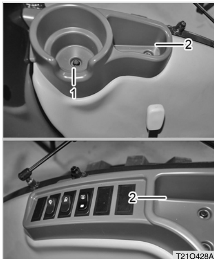
(1) Becherhalter (2) Ablage
