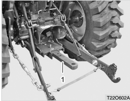
(1) Zugvorrichtung
