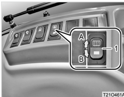
(1) Heckscheibenheizungsschalter (A) EIN (B) AUS
