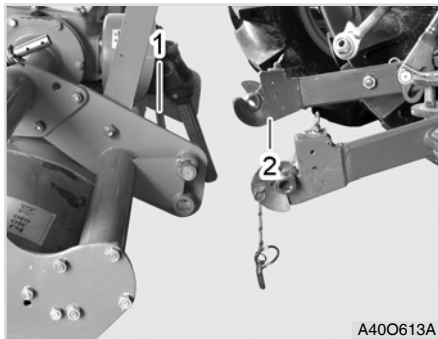
(1) Gerätehalterung (2) Gerätestift
