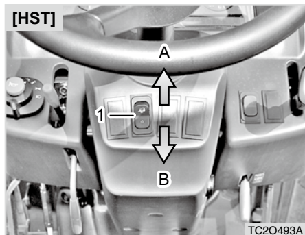
(1) Kontrollschalter Zapfwellen-Geschwindigkeitsregler
