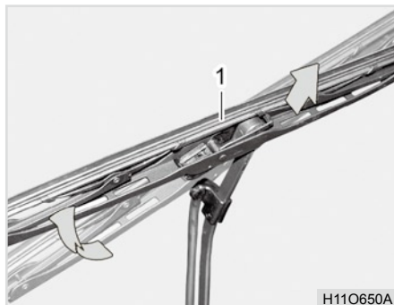
(1) Wischerblatt
