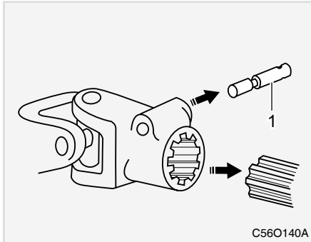
(1) Sperrstift
