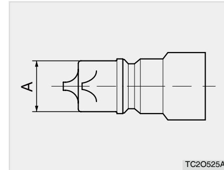
(A) Durchmesser
