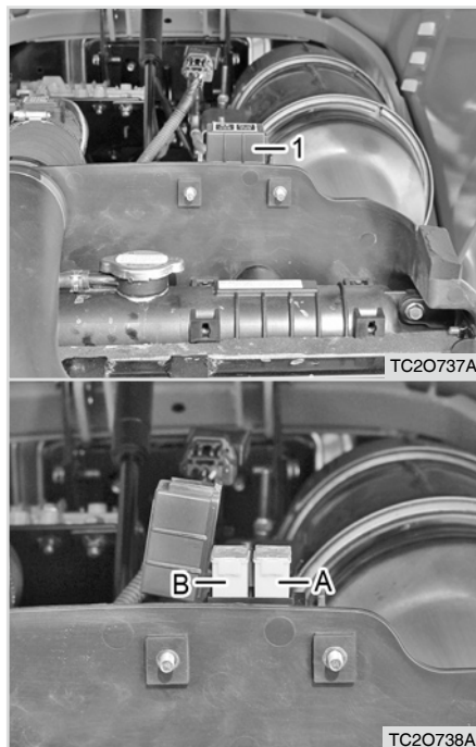
(1) Hauptsicherung
