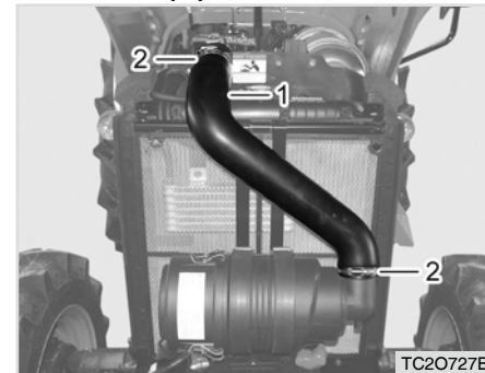
(1) Luftleitungsschlauch
