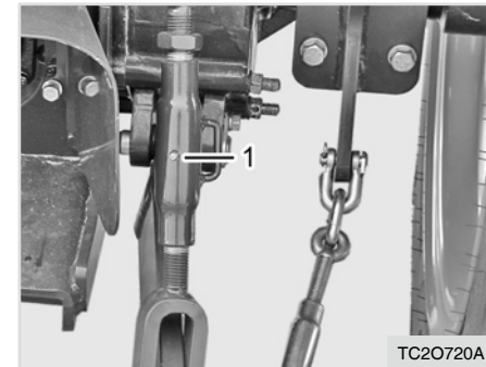
(1) Hebestange
