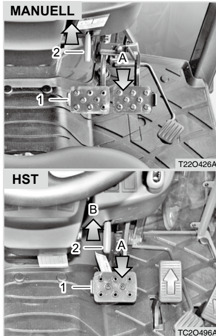
(1) Parkbremshebel (A) Durchdrücken (2) Bremspedal (B) Lösen
