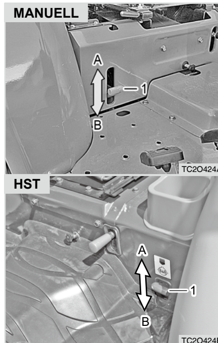
(1) Pedal Differentialsperre (A) Loslassen um zu deaktivieren (B) Verriegeln
