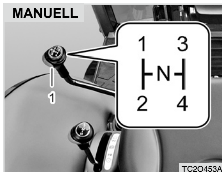
(1) Hauptgangschaltthebel
