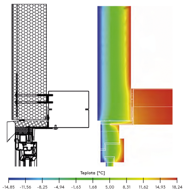
Nadpraží – okno v lici fasády
