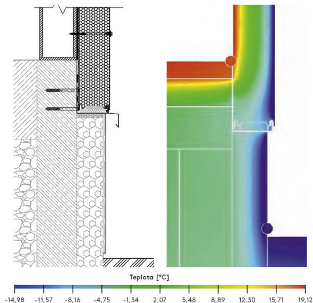
Sokl – podlaha vysoko nad úrovní UT
