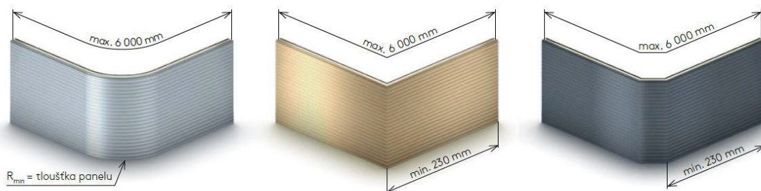
Horizontálně kladené panely
