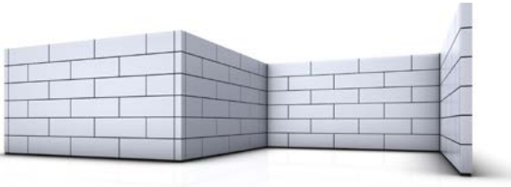
2. Poziomy z przesunięciem - symetryczny
