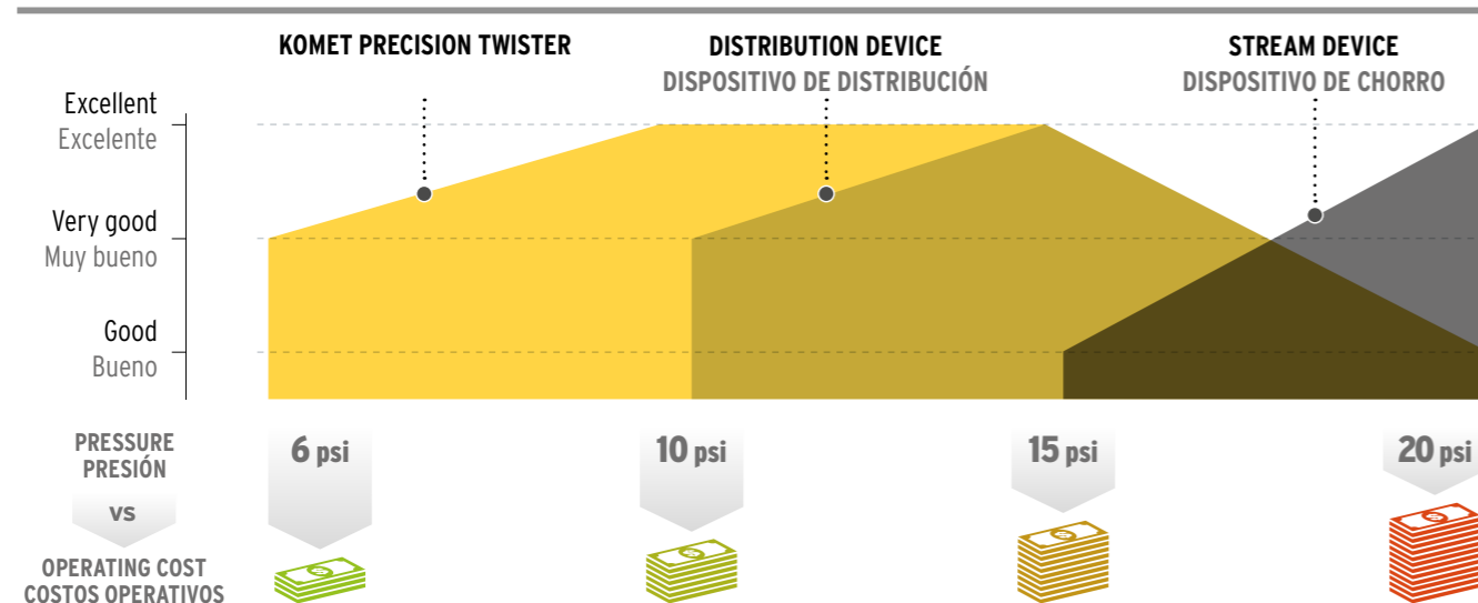
Sprinkler Device Efficiencies / Eficiencia de los dispositivos
