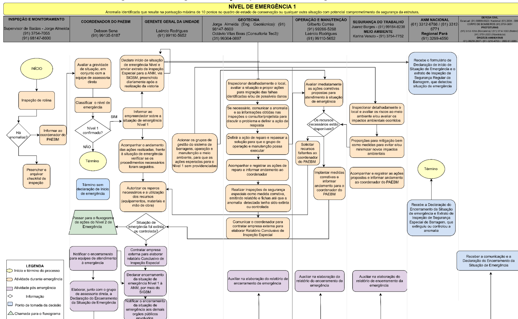
Figura 6-1 – Fluxograma de Ações para Nível de Emergência 1 da Bacia BCA.
