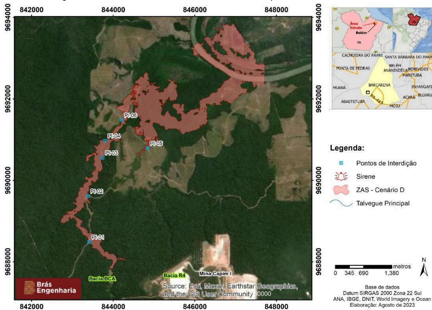
Figura 20-5 – Pontos de Encontro, Sirene, Pontos de Bloqueio e Cadastros – Bacia BCA.
