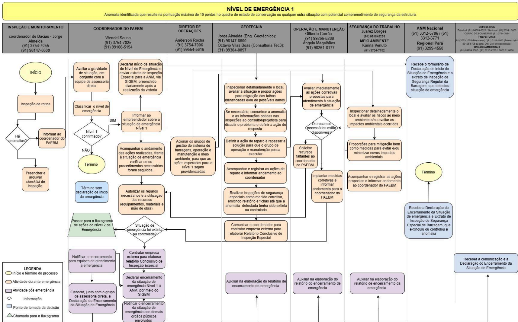
Figura 6-1 – Fluxograma de Ações para Nível de Emergência 1 da Bacia 6B.
