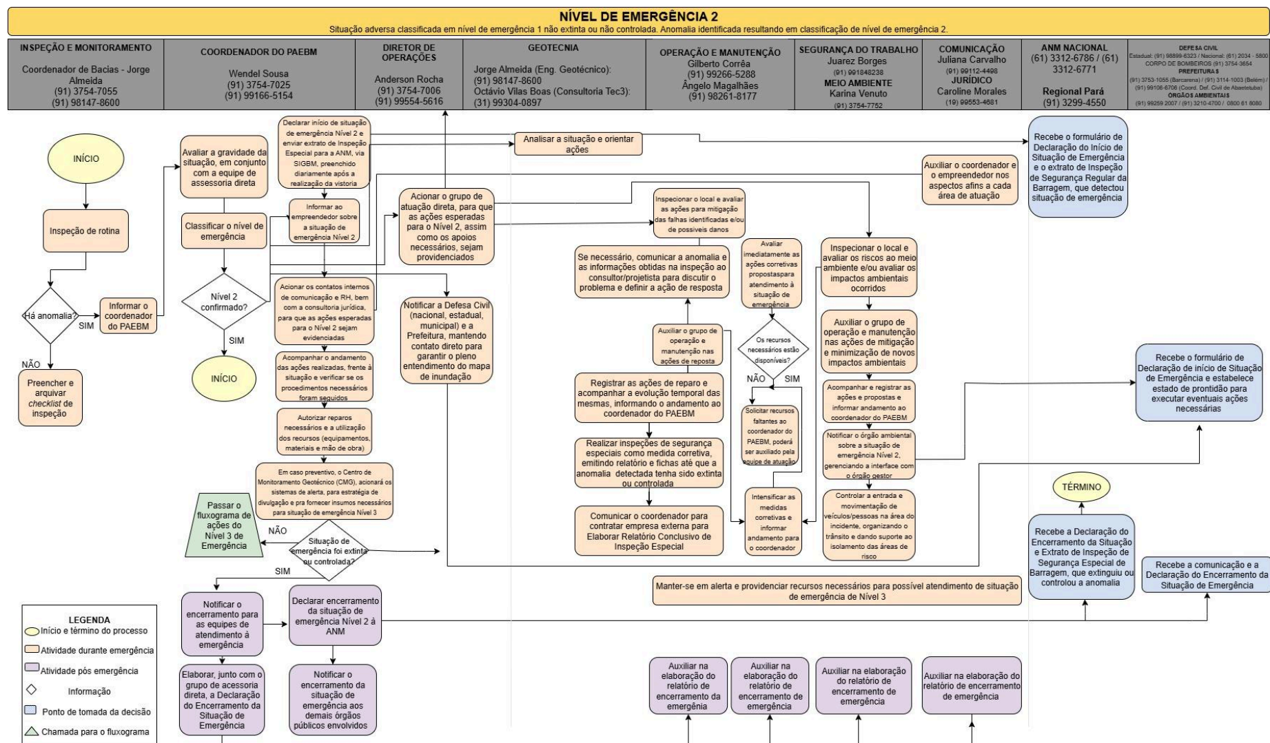
Figura 20-2 – Fluxograma de Ações para Nível de Emergência 2 da Bacia 6B.
