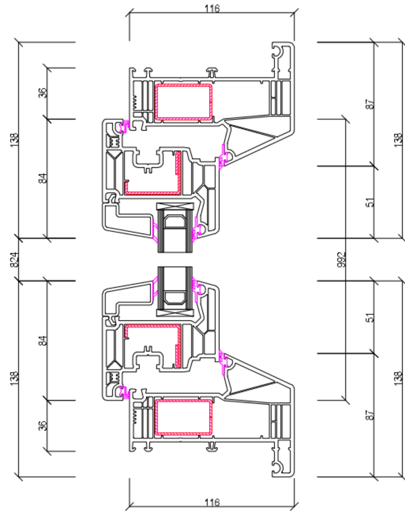
Doorsnede S2, M 5:1
