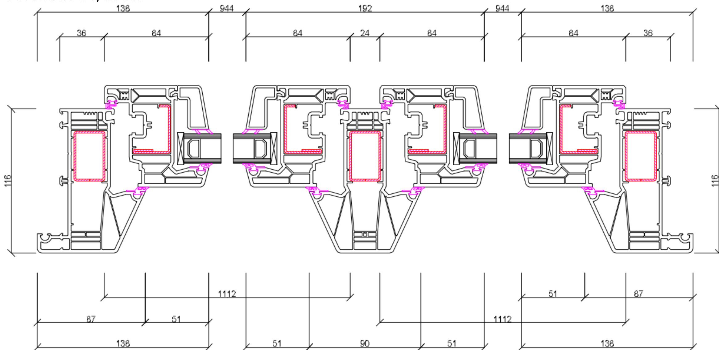
Doorsnede S1, M 5:1
