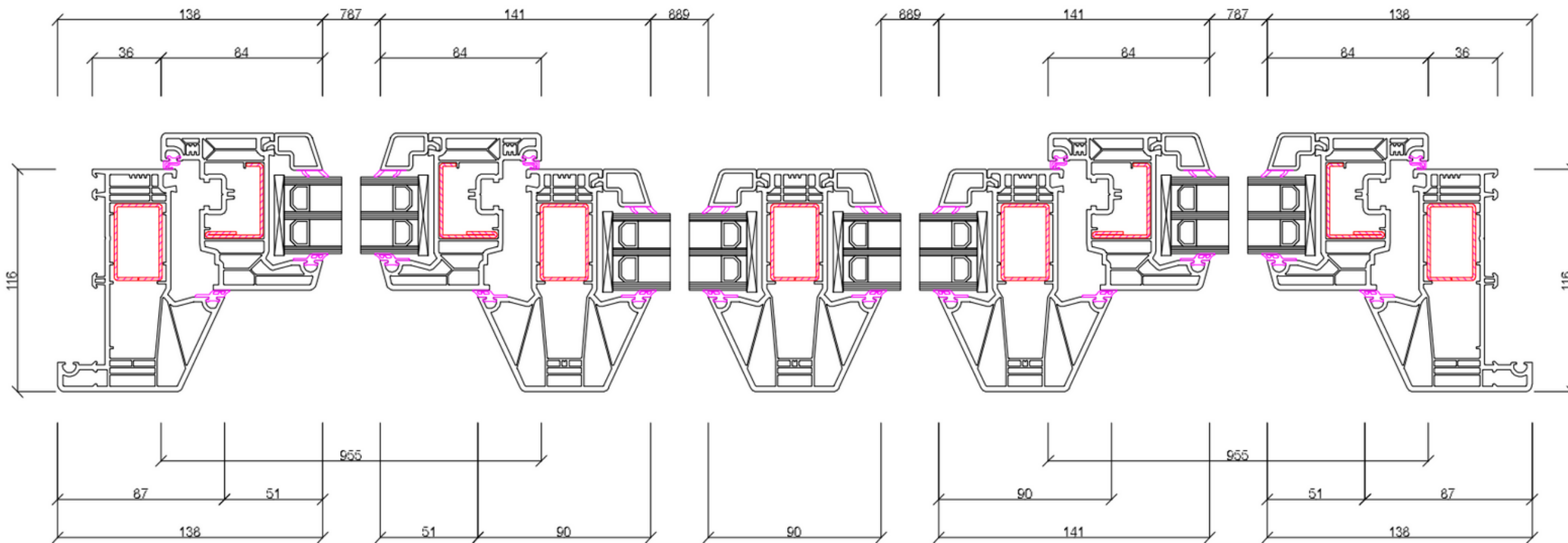
Doorsnede S1, M 5:1
