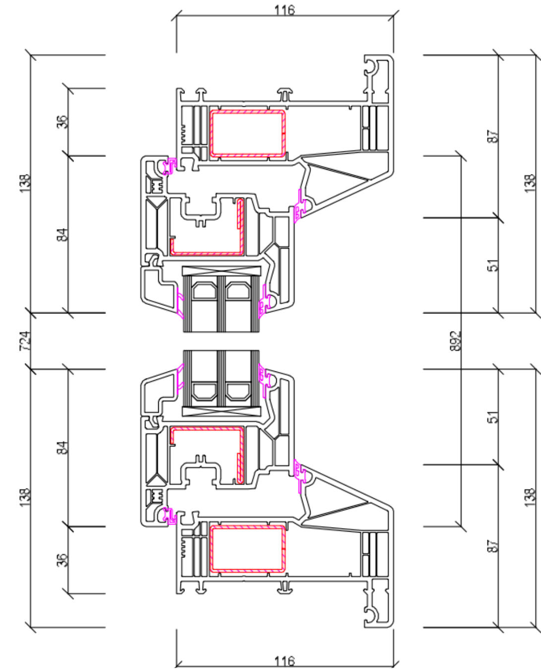
Doorsnede S2, M 5:1
