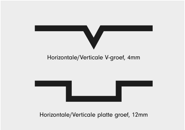
Groefmogelijkheden
