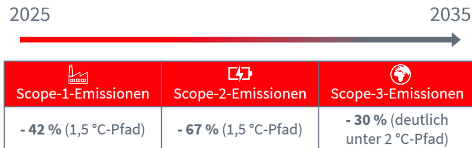
Abbildung 8: THG-Reduktionspfad bis 2035
