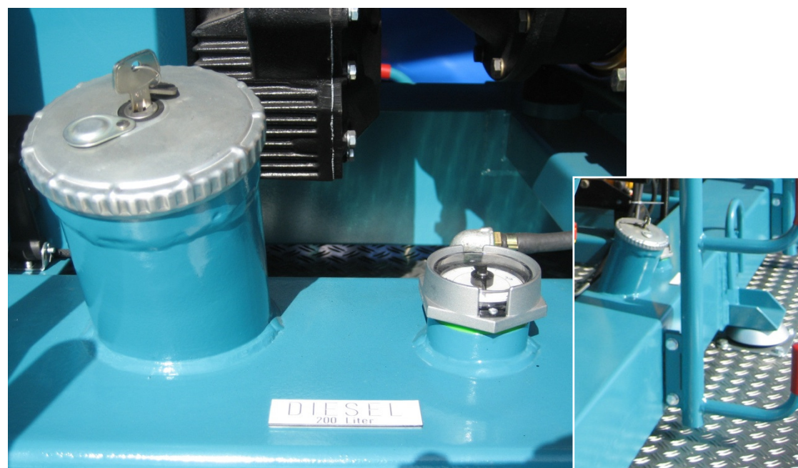
Tank integriert im Grundrahmen montiert, auf schwingungsdämpfenden Füßen mit Füllstandsanzeige
