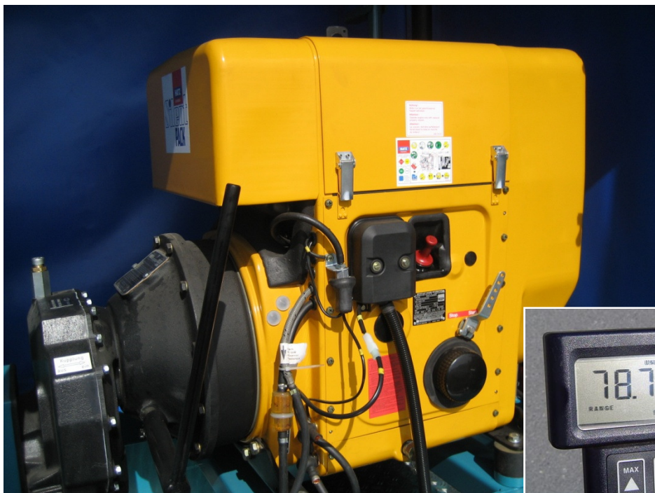
Lärmgekapselter Motor (Hatz) ca. 90 dB(A)
