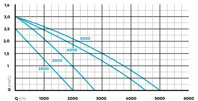
OPTIMAX 2000-5000
