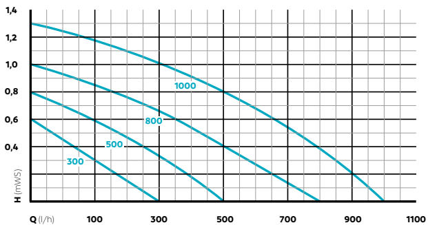
OPTIMAX 300-1000
